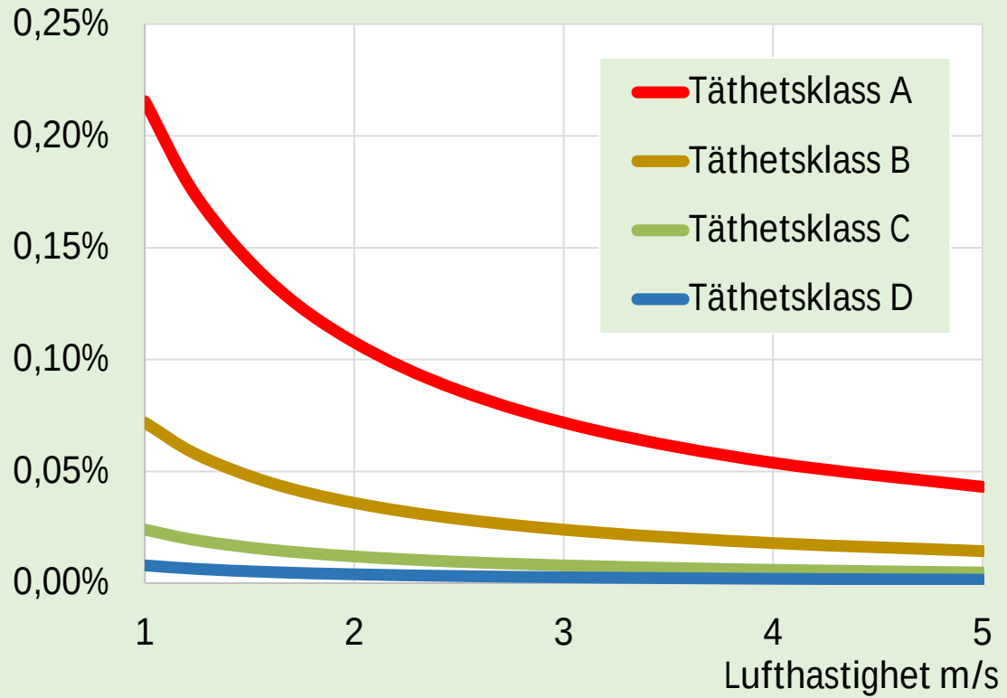
Läckflöde/Kanalflöde, Ø1000 mm, 100 Pa
