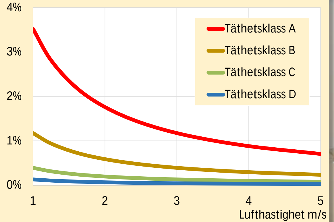
Läckflöde/Kanalflöde, Ø125 mm, 300 Pa
